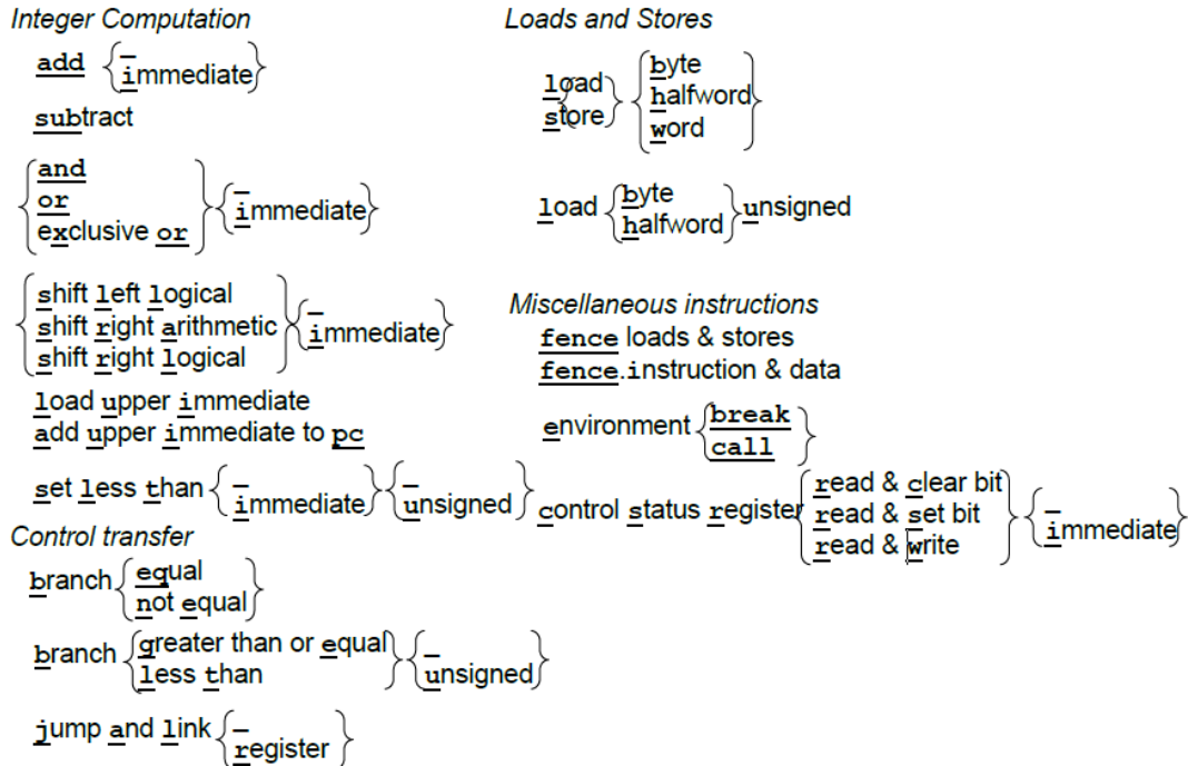
图 2.1: RV32I 指令图示。把带下划线的字母从左到右连接就组成了 RV32I 指令。花括号 {} 表示集合中垂直方向上的每个项目都是指令的不同变体。集合中的下划线_意味着不包含这个字母的也是一个指令名称。例如，左上角附近的符号表示以下六个指令：and, or, xor, andi, ori, xori。
