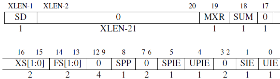
图 10.9: sstatus CSR。sstatus 是 mstatus (图 10.4) 的一个子集, 因此它们的布局类似。SIE 和 SPIE 中分别保存了当前的和异常发生之前的中断使能, 类似于 mstatus 中的 MIE 和 MPIE。RV32 的 XLEN 为 32, RV64 为 40。(来自 [Waterman and Asanovic 2017] 中的图 4.2; 有关其他域的说明请参见该文档的第 4.1 节。)
